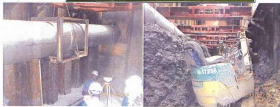
左が使用中の下水道管φ450mmです。右側の掘削機のあるところに新設管を置いた後、使用中の管を取り壊します。
