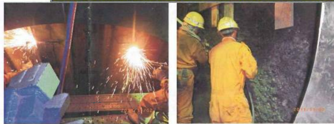
11月4日からシールド機の掘進を始めて、6日に機械全体が地山に貫入した
