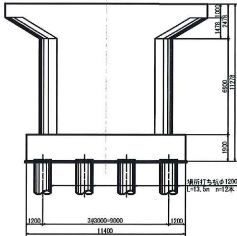
橋脚
