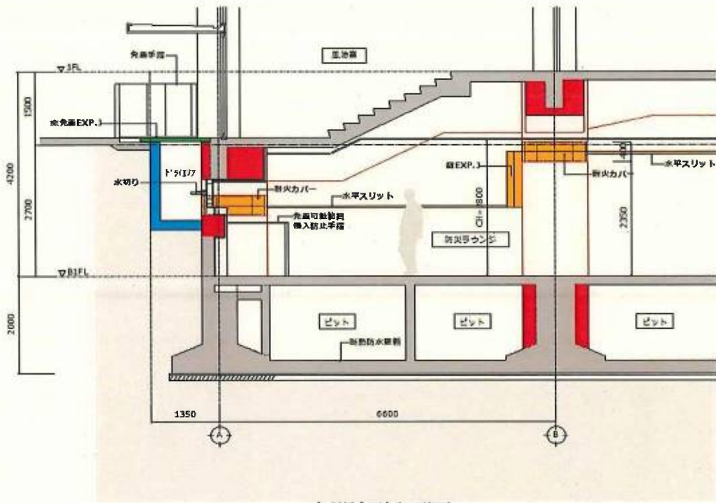
玄関部断面図
