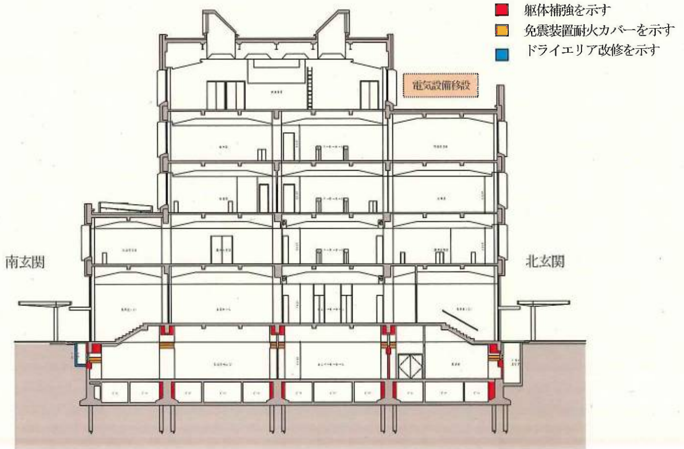
全体断面図
