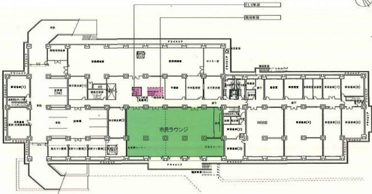
地下1階平面図 (工事完成後)
