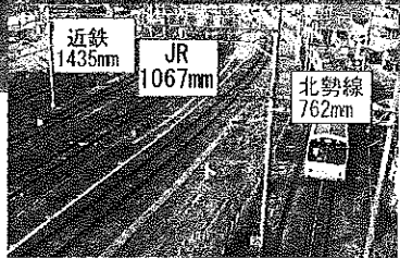
軌道幅が762mmの特殊狭軌(ナローゲージ)
